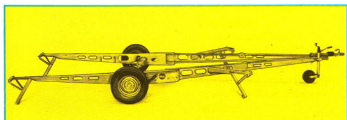
Breitspurfahrwerk mit Einzelradaufhängung.
