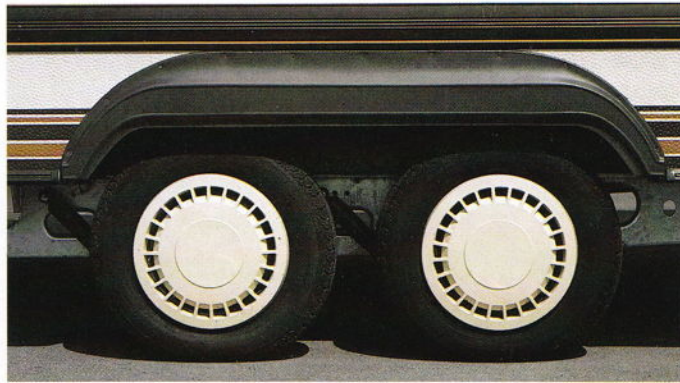
Tandemachse bei den Modellen 580, 680 und 690. Breitspurfahrwerk mit Einzerradaufhängung (Westeurop. SR-Markenreifen).
